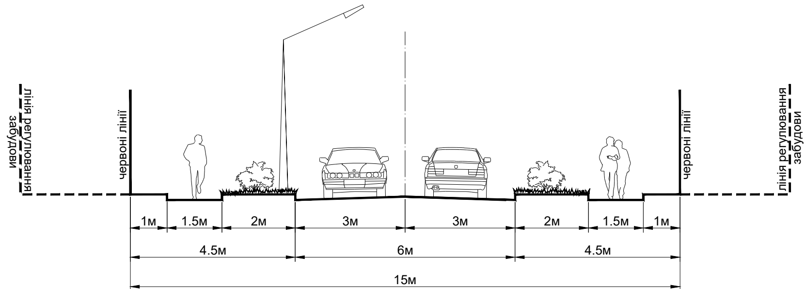
ПРОФІЛЬ І-І
